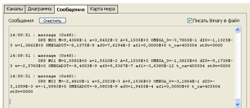
Рис. 15. Отображение загрузки альманаха во вкладке «Сообщения»
