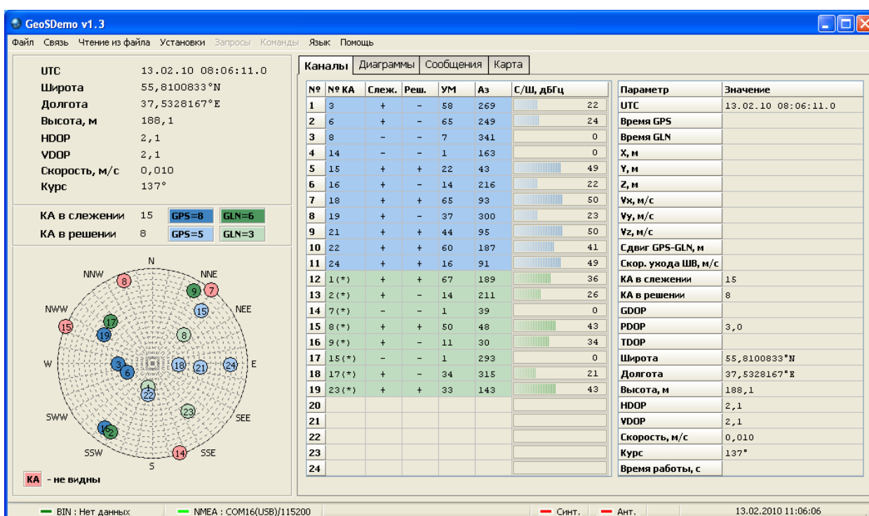
Рис. 9. Основное окно программы GeoSDemo® при работе по NMEA протоколу
