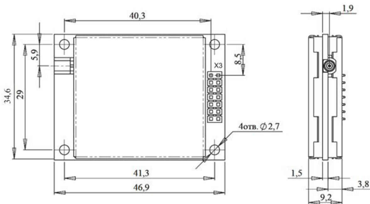
рис. 2. Габаритно-присоединительные размеры приемника
