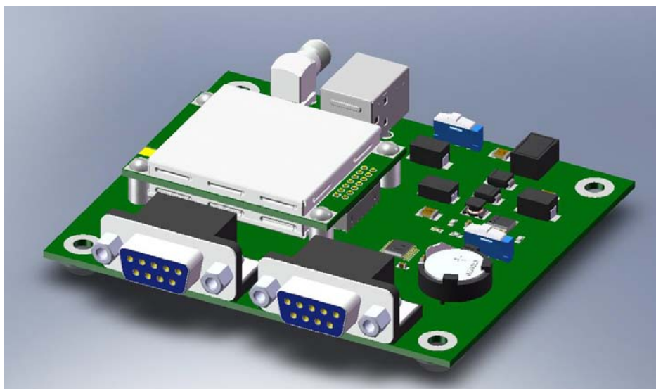
Рис. 27. Установка приемника на плату коммутации
