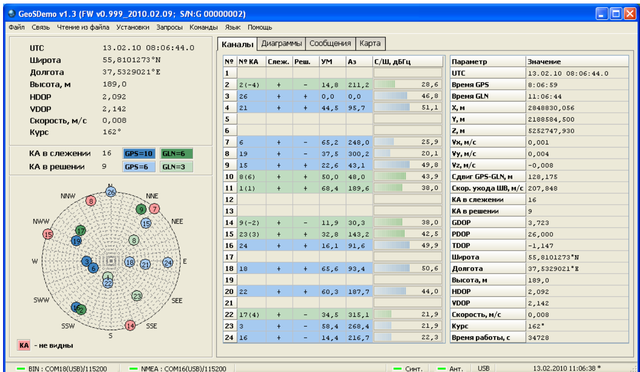
Рис. 8. Основное окно программы GeoSDemo® при работе по бинарному протоколу
