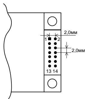
Рис. 1. Разводка выходного НЧ соединителя
