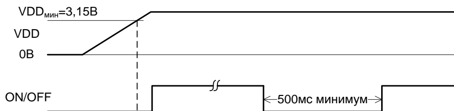
Рис. 4. Временная диаграмма управления включением/выключением приемника
