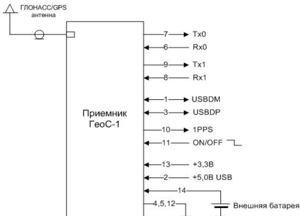
Рис. 3. Типовая схема подключения приемника
