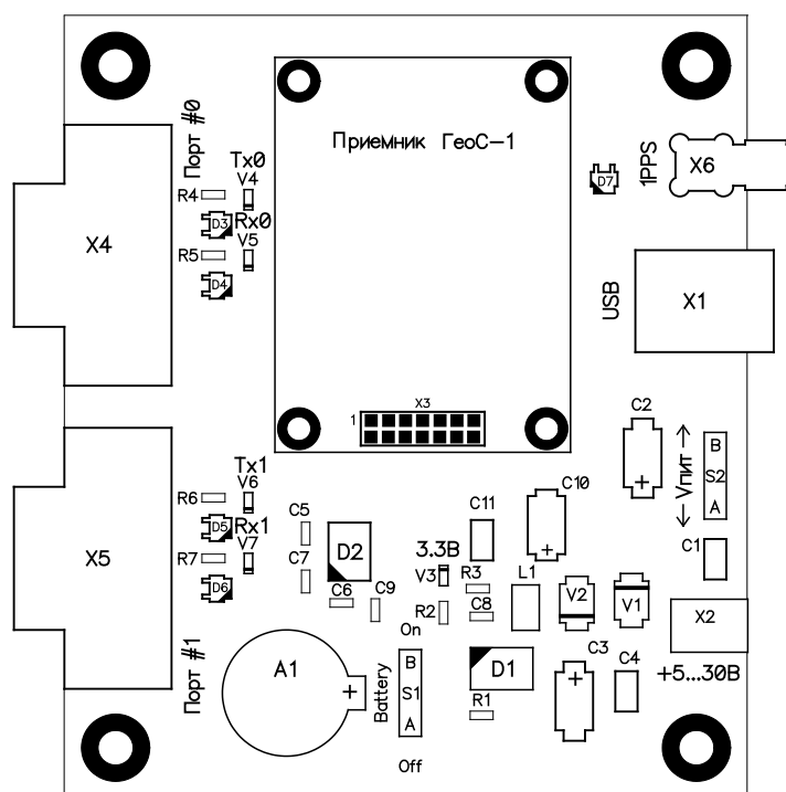
Рис. 26. Внешний вид платы коммутации ГеоС-1
