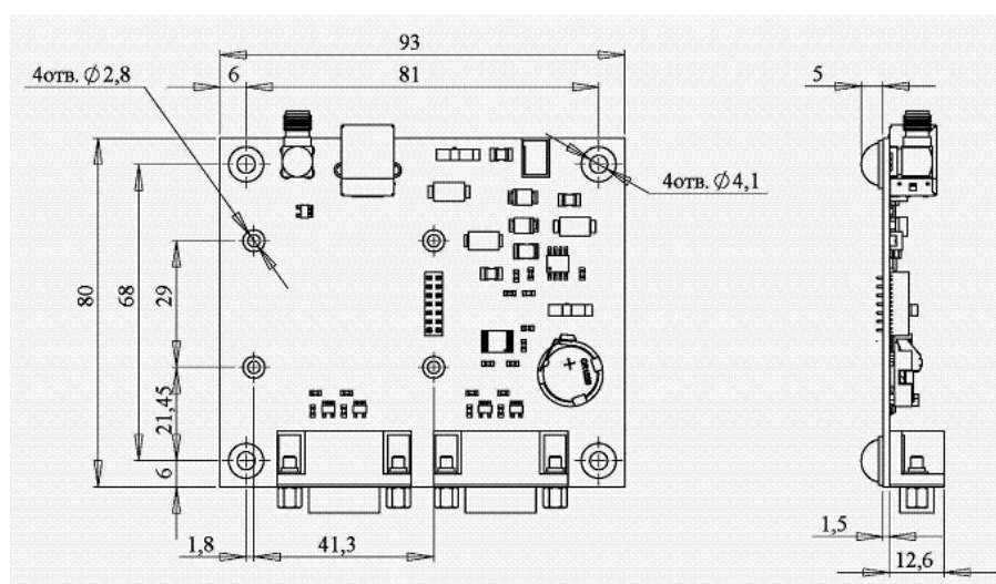
Рис. 28. Габаритно-присоединительные размеры платы коммутации
